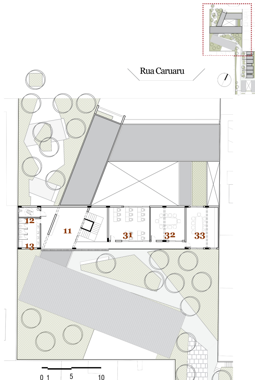
PLANTA BAIXA 2º PAVIMENTO AMPLIADA
