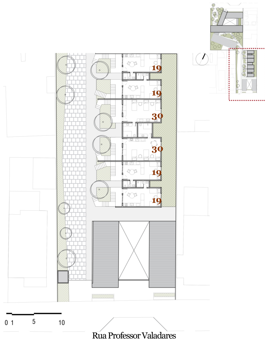
PLANTA BAIXA 1º PAVIMENTO AMPLIADA
