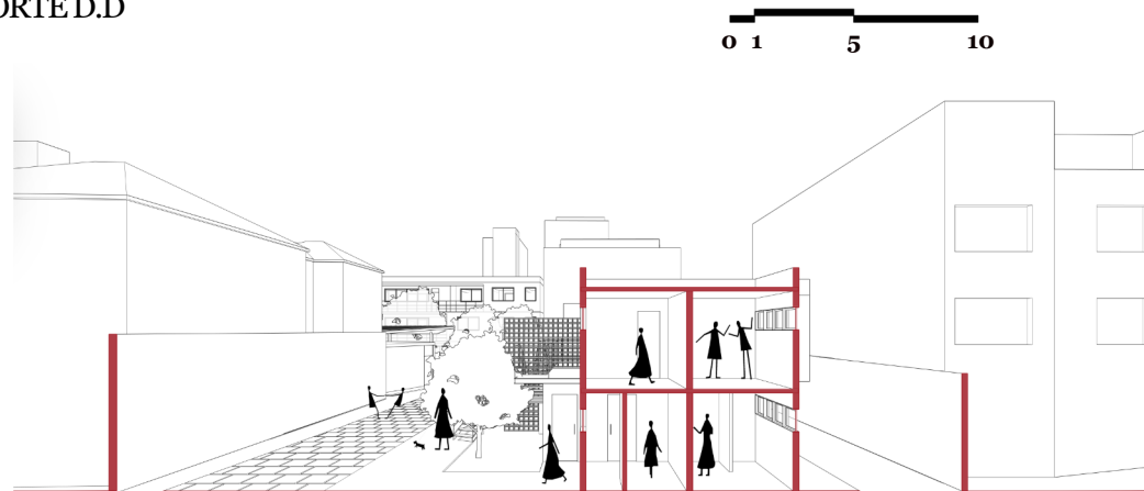
CORTE E.E
